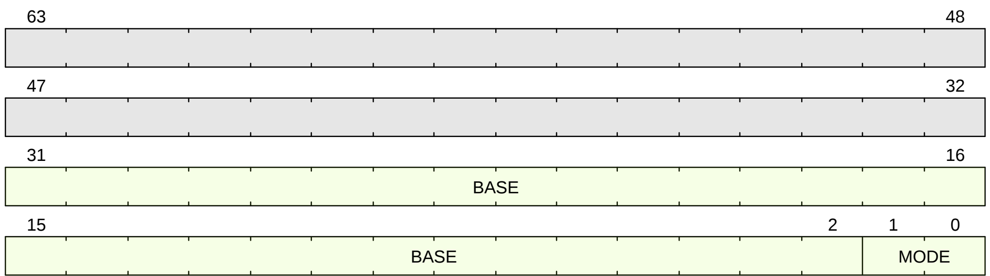
Figure 17. mtvec format
