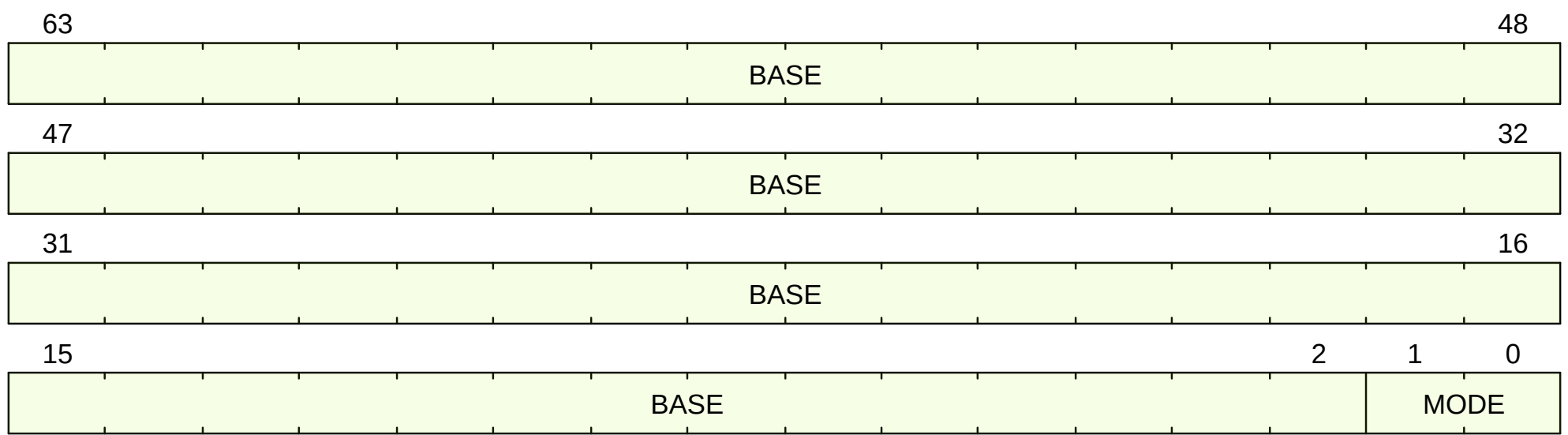
Figure 50. stvec format
